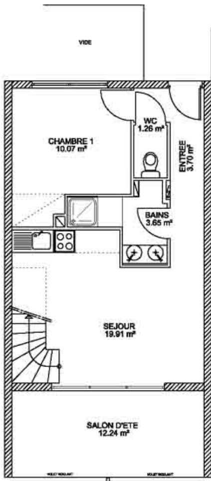
NIVEAU HAUT
